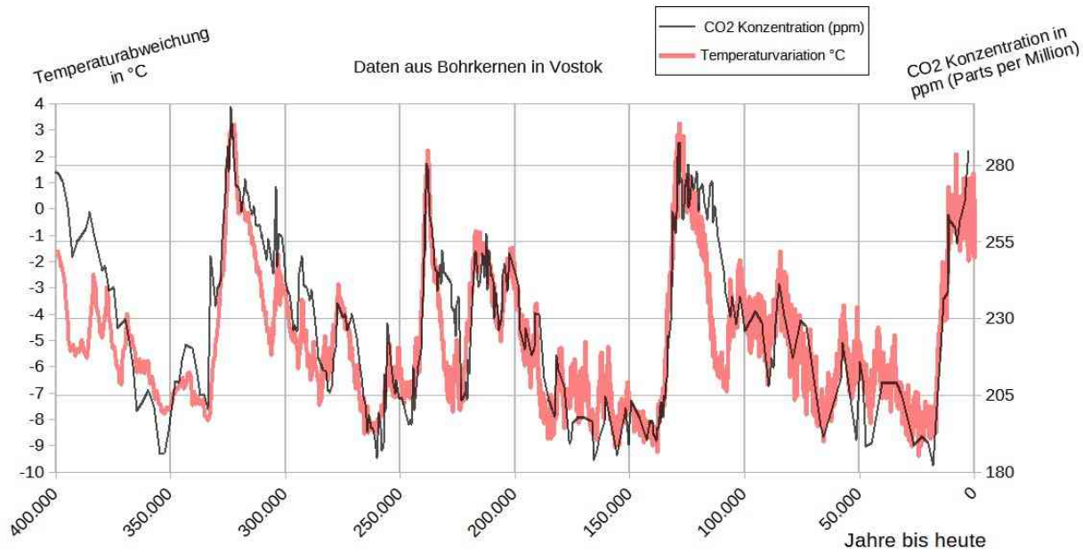
Quelle: Diagramm auf Basis des Datensatzes der Vostok-Eisbohrkerne
