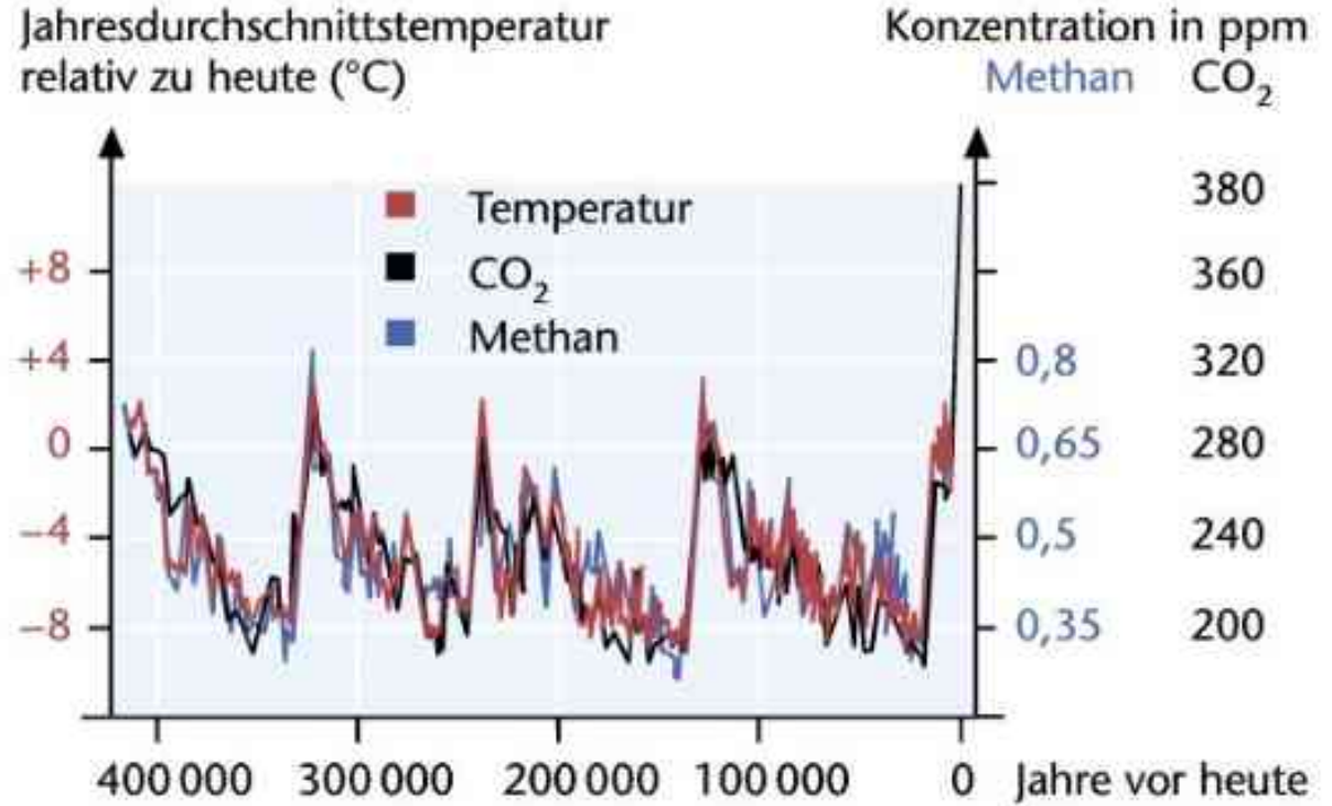
3 Temperaturschwankungen und Treibhausgas-Konzentrationen der letzten 400 000 Jahre
