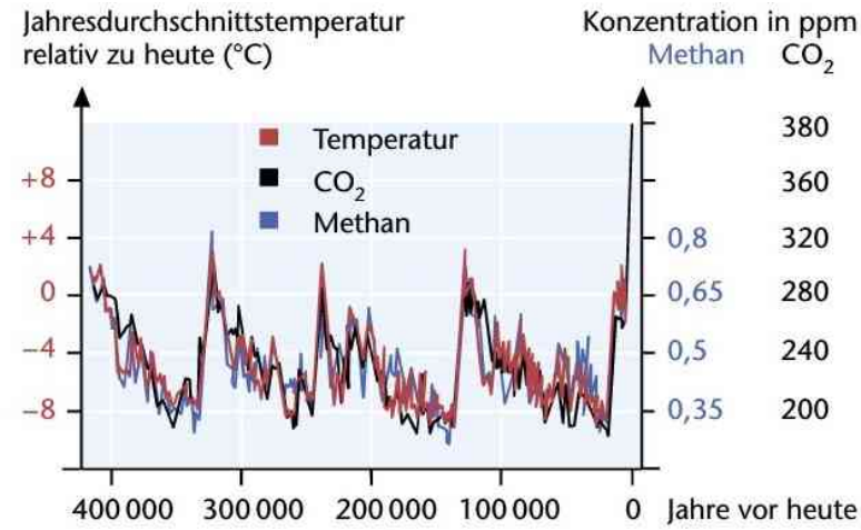
3 Temperaturschwankungen und Treibhausgas-Konzentrationen der letzten 400 000 Jahre
